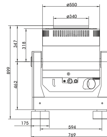
S 56280/LS-340 (Beispielzeichnung) Maße in mm
